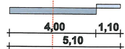
profil existent Aleea Taifunului
