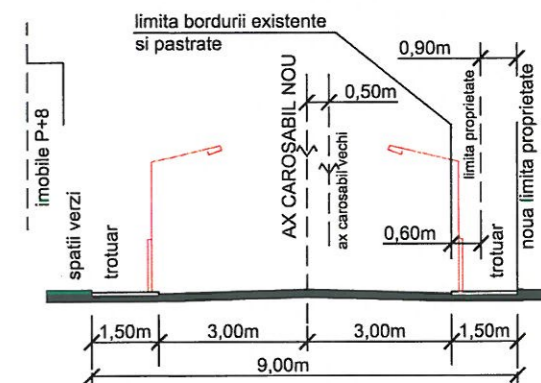
PROFIL propus STR. DANUBIU - Sc: 1:200
