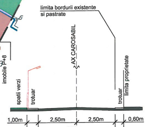
PROFIL existent STR. DANUBIU - Sc: 1:200
