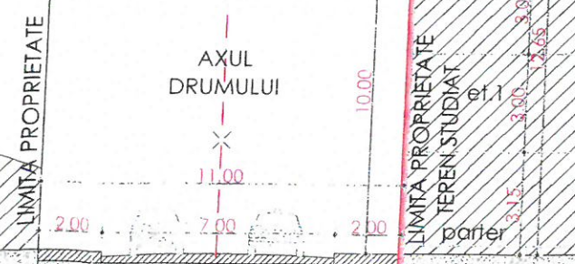
SECȚIUNE S-S STR.LT.COL.PAPAZOGLU SCARA 1:200
