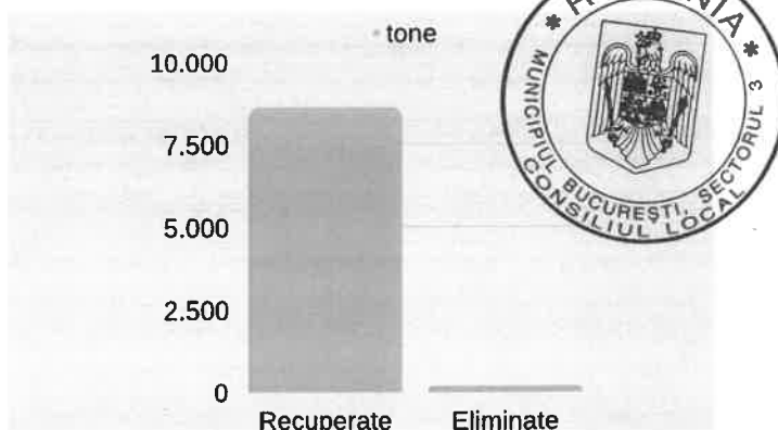
Graf. 2: Deșeuri provenite din construcții, Ian-Dec 2021
