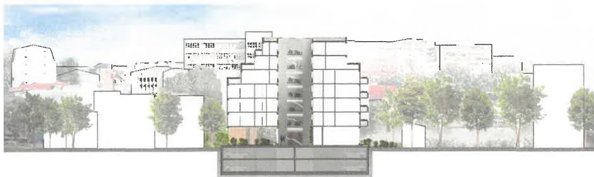
SECȚIUNE CARACTERISTICĂ, PRIVIND RELAȚIA DINTRE ÎNĂLȚIMEA FONDULUI CONSTRUIT EXISTENT ȘI CLĂDIREA PROPUȘĂ
