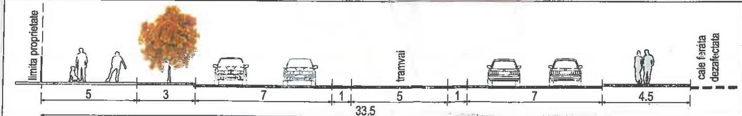
Profil A-A - Bdul Basarabia - existent, sc. 1:200
