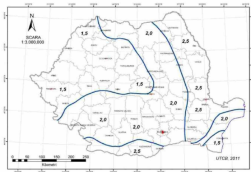
Figura 3.1 Zonarea valorilor caracteristice ale încărcării din zapada pe sol S_s , kN/m 2 , pentru altitudini A = 1000 m NOTA: Pentru altitudini A > 1000 m valorile S_s se determina cu relațiile (3.1) și (3.2)
