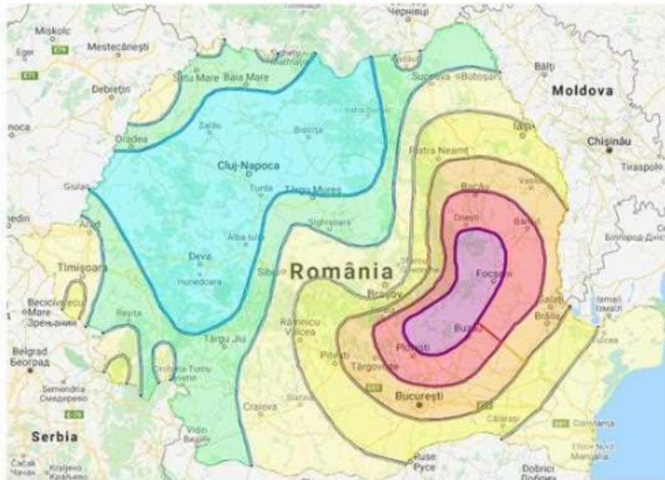
Figura 3.1: Zonarea teritoriului României în termeni de valori de vârf ale accelerăției terenului de proiectare a_g pentru cutremure având intervalul mediu de recurență IMR= 225 ani și 20% probabilitate de depășire în 50 de ani
