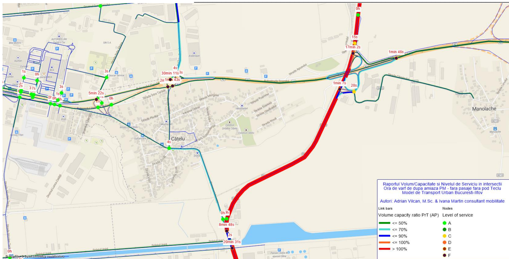
Fig. 30 – Întârzieri si Nivelul de Serviciu in intersectii - Raportul Volum/Capacitate pe bara dintre intersectii - situația fără pasaje fără pod Teclu, ora de vârf de după amiaza PM, detaliu Est
