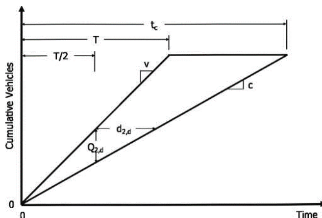
Fig. 79 – Acumularea sosirilor in intersecție si plecările pe durata perioadei suprasaturate de trafic
