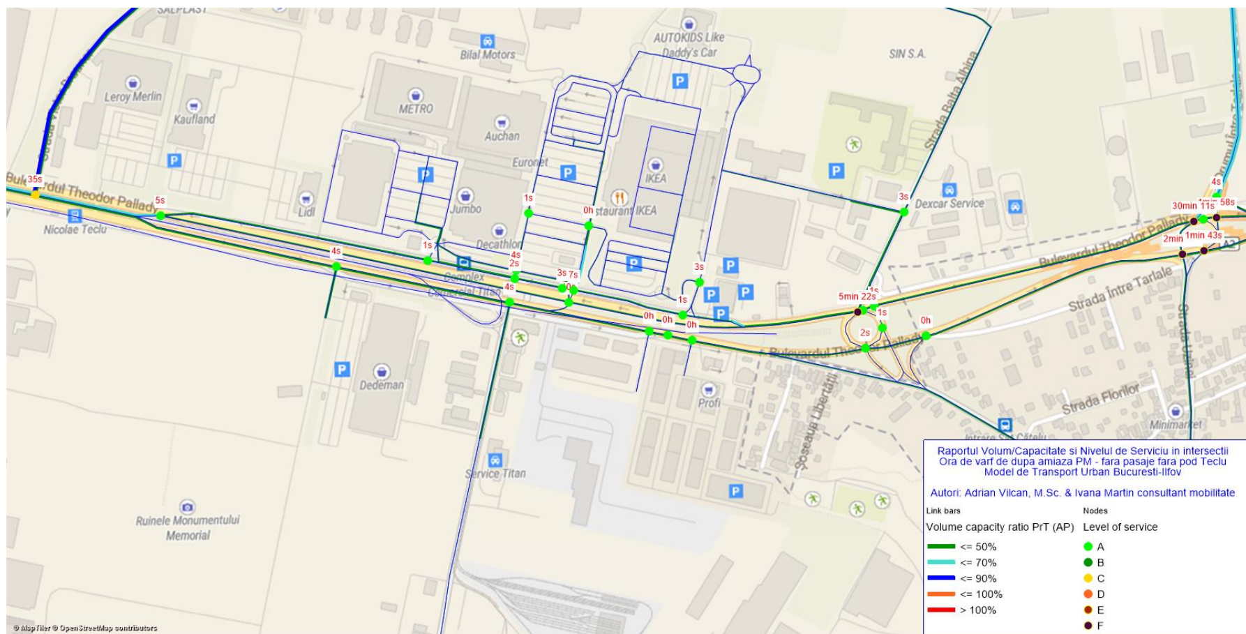
Fig. 29 – Întârzieri și Nivelul de Serviciu în intersecții - Raportul Volum/Capacitate pe bara dintre intersecții - situația fără pasaje fără pod Teclu, ora de vârf de după amiaza PM, detaliu Vest
