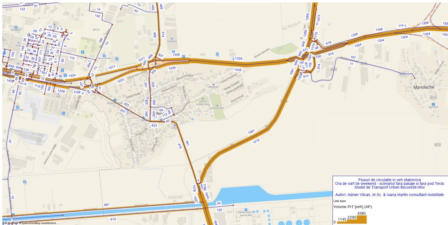
Fig. 63 – Debite de trafic - situația fără pasaje fără pod Teclu, ora de vârf de sâmbătă - veh/ora, detaliu Est
