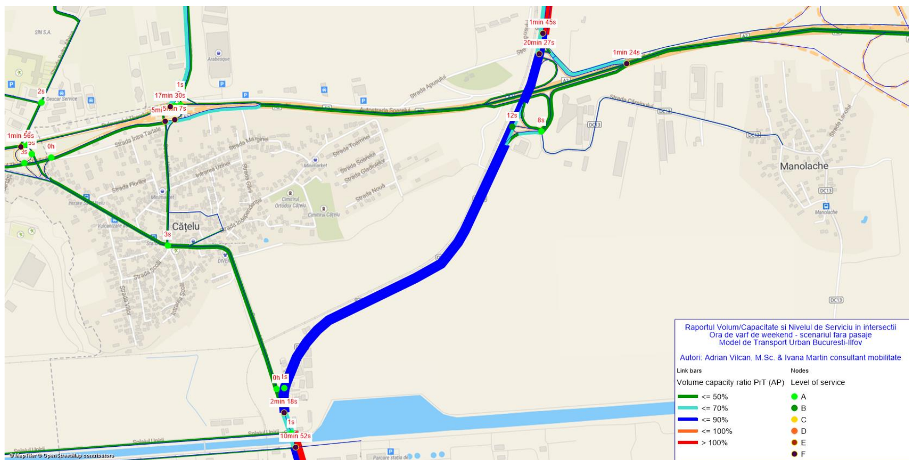
Fig. 72 – Întârzieri si Nivelul de Serviciu in intersecții - Raportul Volum/Capacitate pe bara dintre intersecții - situația fără pasaje, ora de vârf de sâmbătă, detaliu Est
