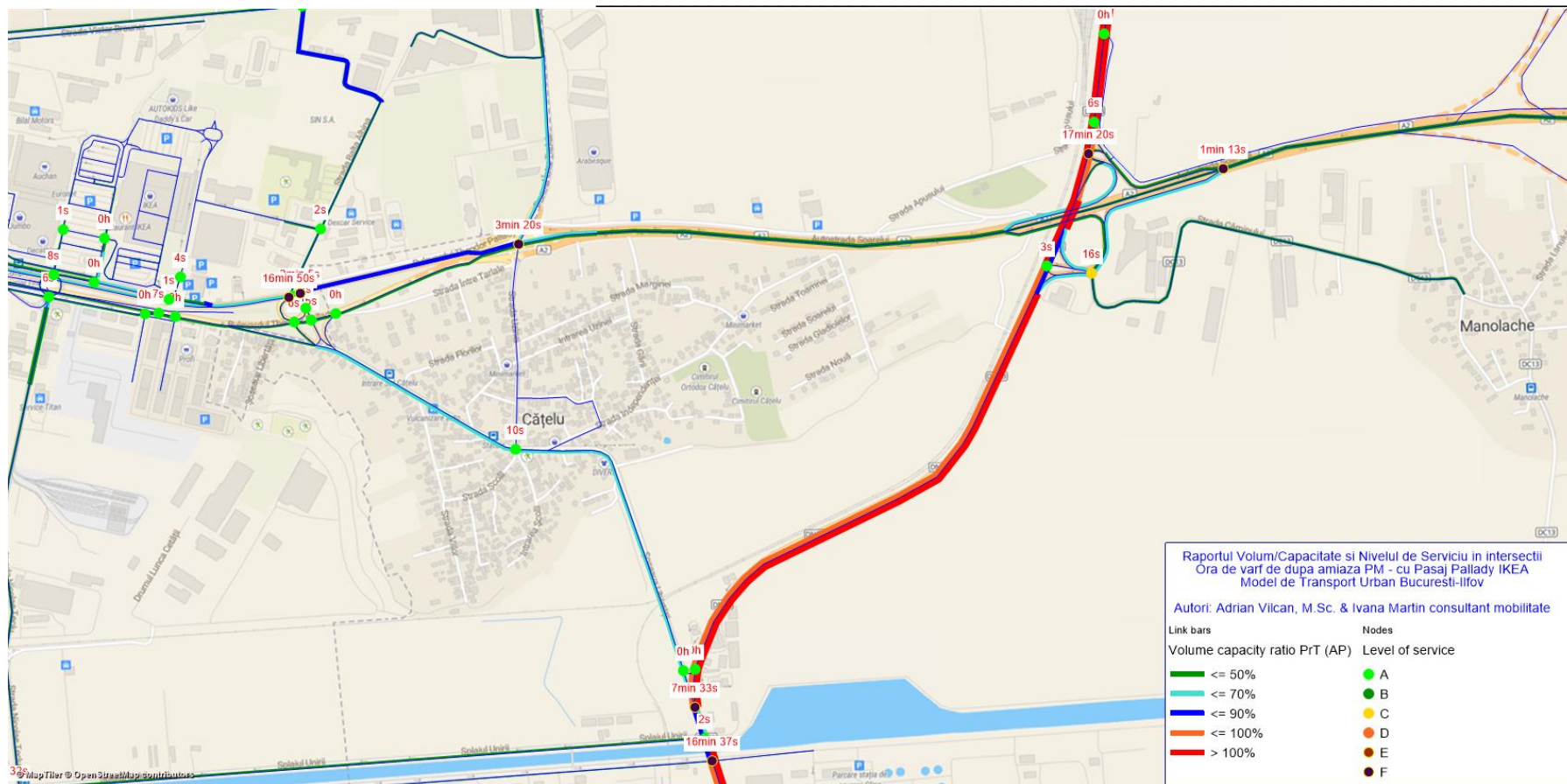
Fig. 54 – Întârzieri si Nivelul de Serviciu in intersectii - Raportul Volum/Capacitate pe bara dintre intersectii - scenariul cu pasaj IKEA, ora de vârf de după amiaza PM, detaliu Est
