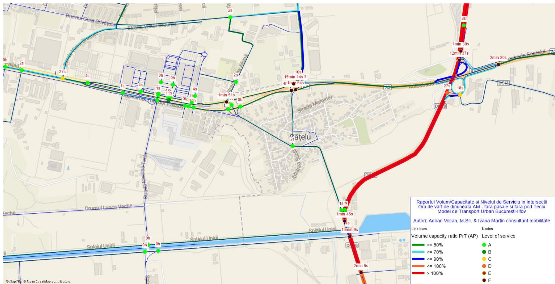
Fig. 22 – Întârzieri si Nivelul de Serviciu in intersectii - Raportul Volum/Capacitate pe bara dintre intersectii - situația fără pasaje fără pod Teclu, ora de vârf de dimineața AM, vedere de ansamblu
