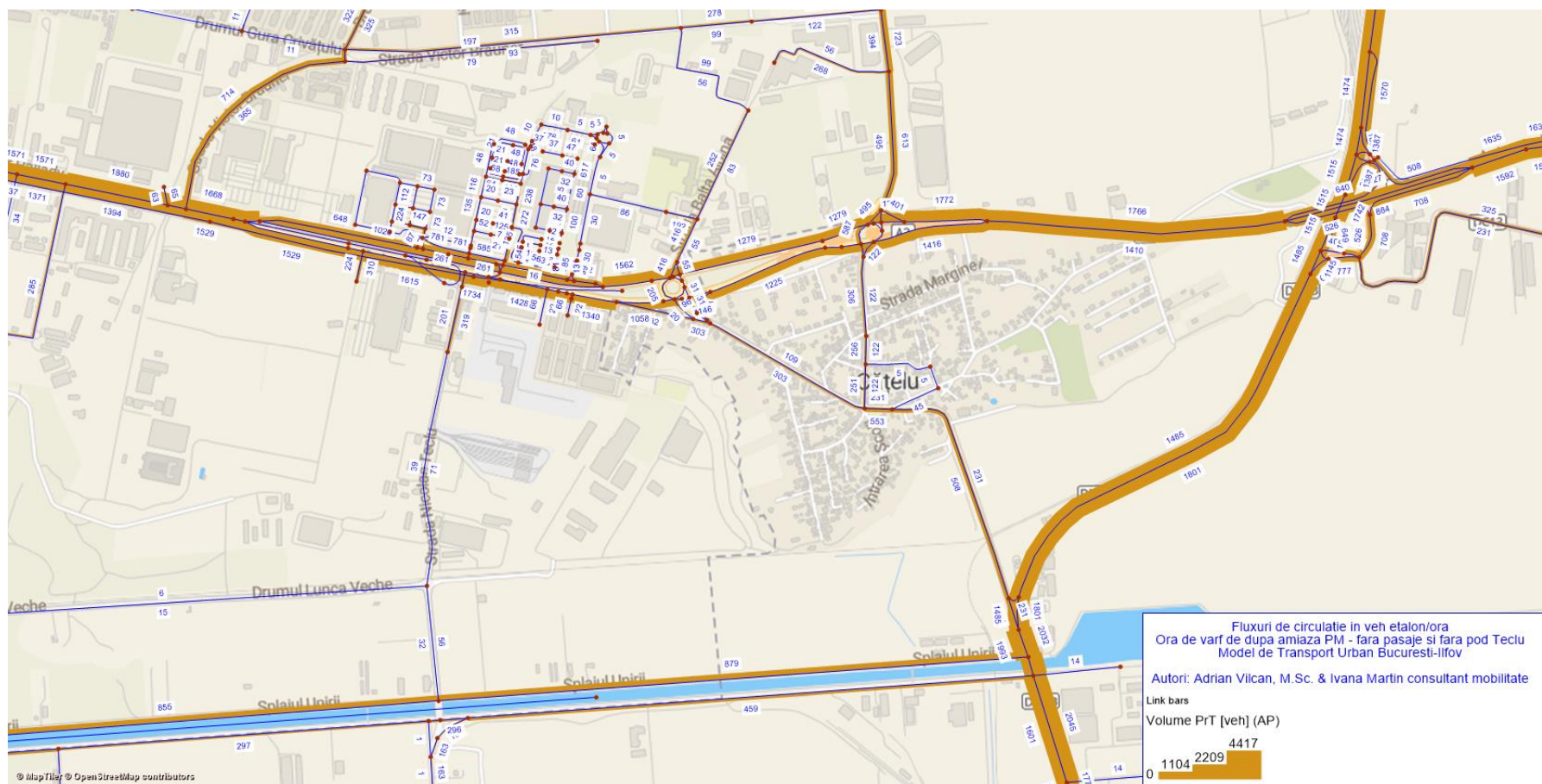
Fig. 25 – Debite de trafic - situația fără pasaje fără pod Teclu, ora de vârf de PM - veh/ora, vedere de ansamblu
