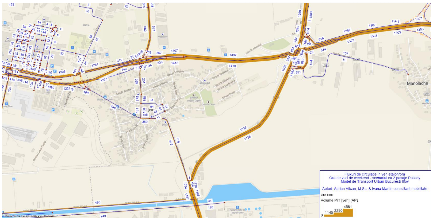
Fig. 57 – Debite de trafic - situația actuală de circulație ora de vârf de sâmbătă - veh/ora, detaliu Est
