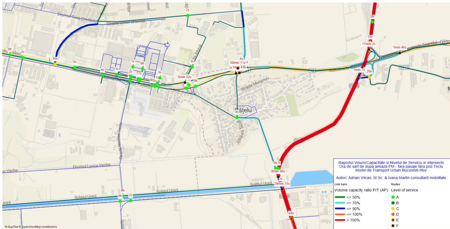
Fig. 28 – Întârzieri și Nivelul de Serviciu în intersecții - Raportul Volum/Capacitate pe bară dintre intersecții - situația fără pasaje fără pod Teclu, ora de vârf de după amiaza PM, vedere de ansamblu
