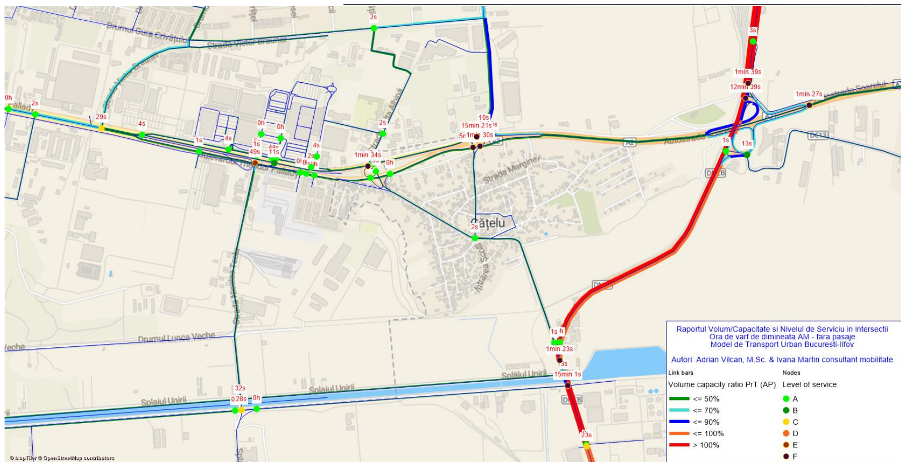
Fig. 34 – Întârzieri si Nivelul de Serviciu in intersectii - Raportul Volum/Capacitate pe bara dintre intersectii - situația fără pasaje, ora de vârf de dimineața AM, vedere de ansamblu
