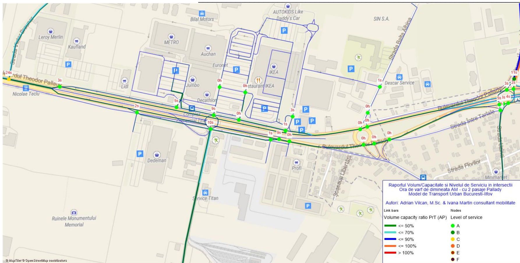
Fig. 11 – Întârzieri si Nivelul de Serviciu in intersectii - Raportul Volum/Capacitate pe bara dintre intersectii - situația actuala de circulație ora de vârf de dimineața AM, detaliu Vest
