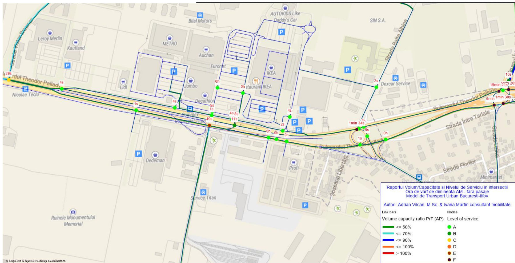
Fig. 35 – Întârzieri si Nivelul de Serviciu in intersectii - Raportul Volum/Capacitate pe bara dintre intersectii - situatia fără pasaje, ora de vârf de dimineata AM, detaliu Vest
