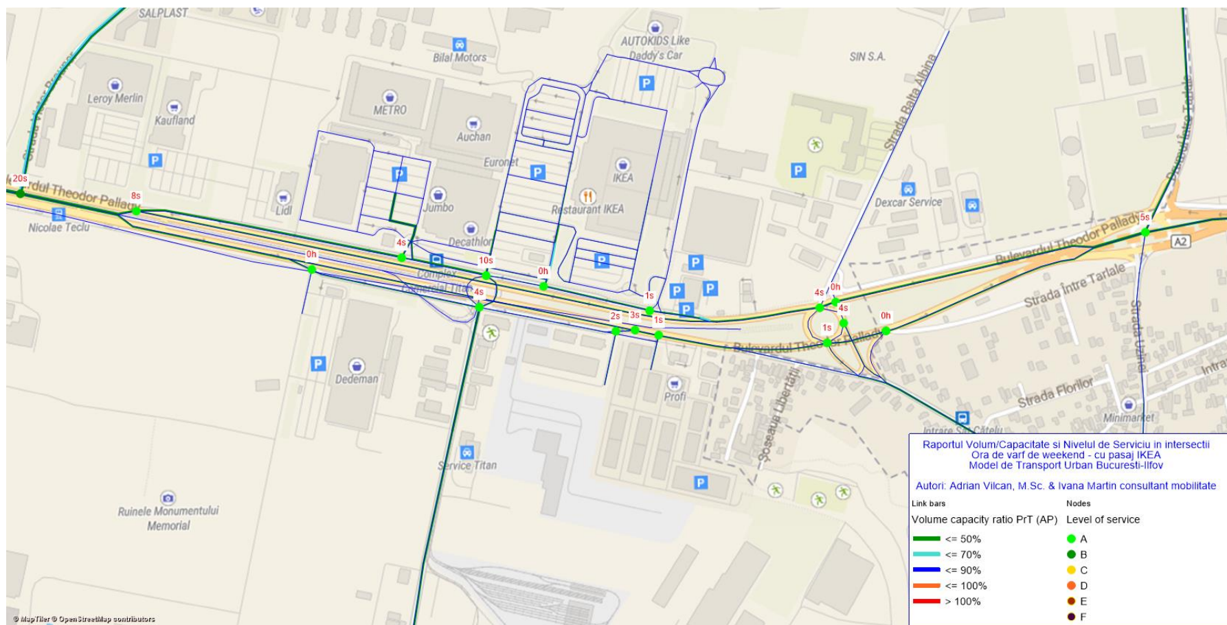
Fig. 77 – Întârzieri și Nivelul de Serviciu în intersecții - Raportul Volum/Capacitate pe bară dintre intersecții - scenariul cu pasaj IKEA, ora de vârf de sâmbătă, detaliu Vest
