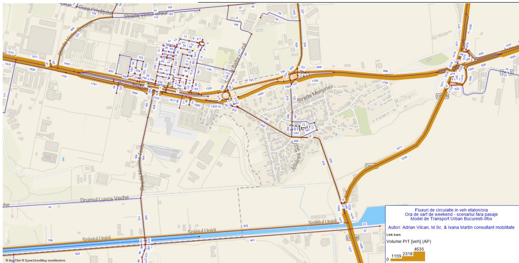
Fig. 67 – Debite de trafic - situația fără pasaje, ora de vârf de sâmbătă - veh/ora, vedere de ansamblu
