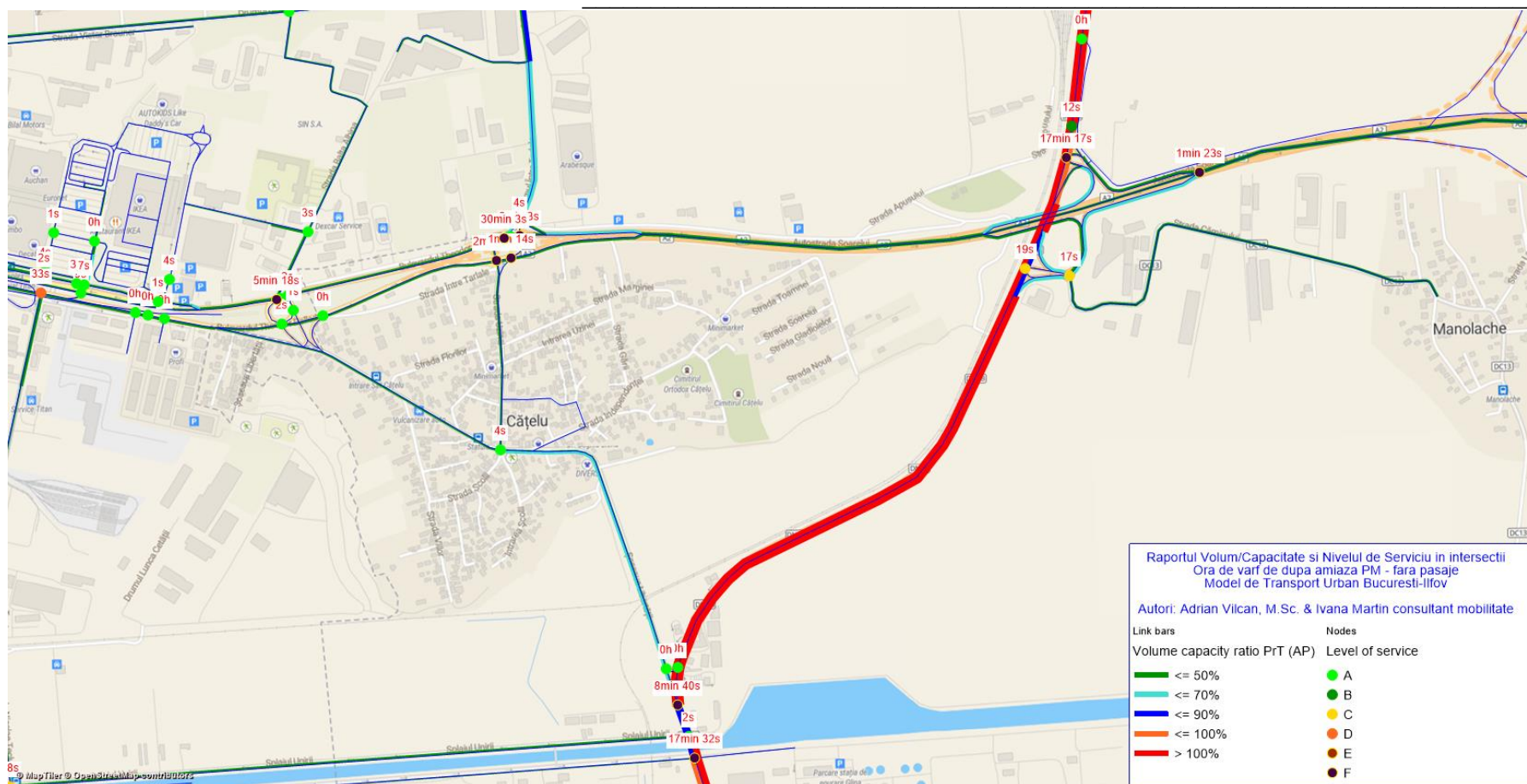
Fig. 42 – Întârzieri si Nivelul de Serviciu in intersectii - Raportul Volum/Capacitate pe bara dintre intersectii - situația fără pasaje, ora de vârf de după amiaza PM, detaliu Est
