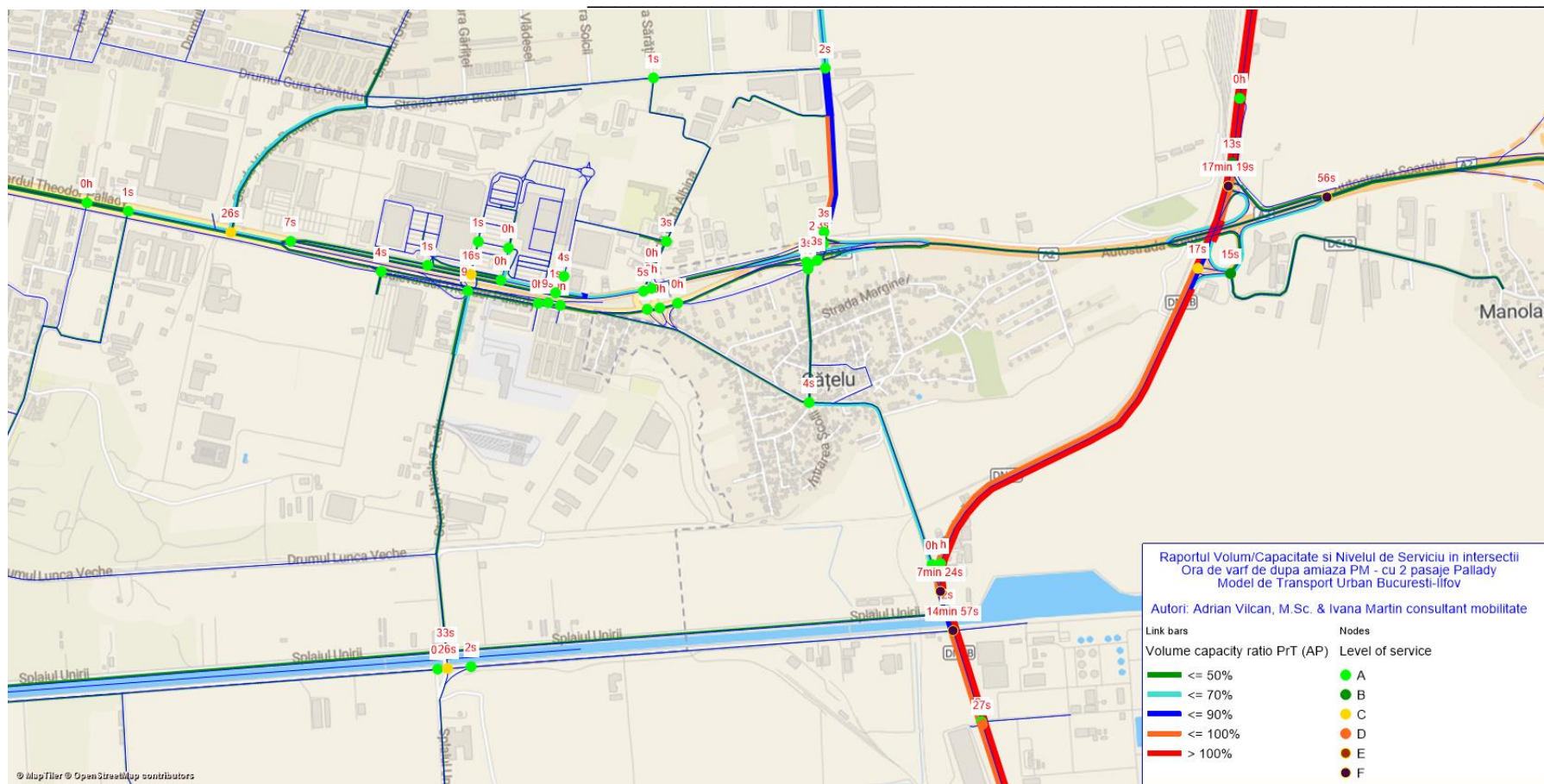
Fig. 16 – Întârzieri și Nivelul de Serviciu în intersecții - Raportul Volum/Capacitate pe bară dintre intersecții - situația actuală de circulație ora de vârf de după amiaza PM, vedere de ansamblu
