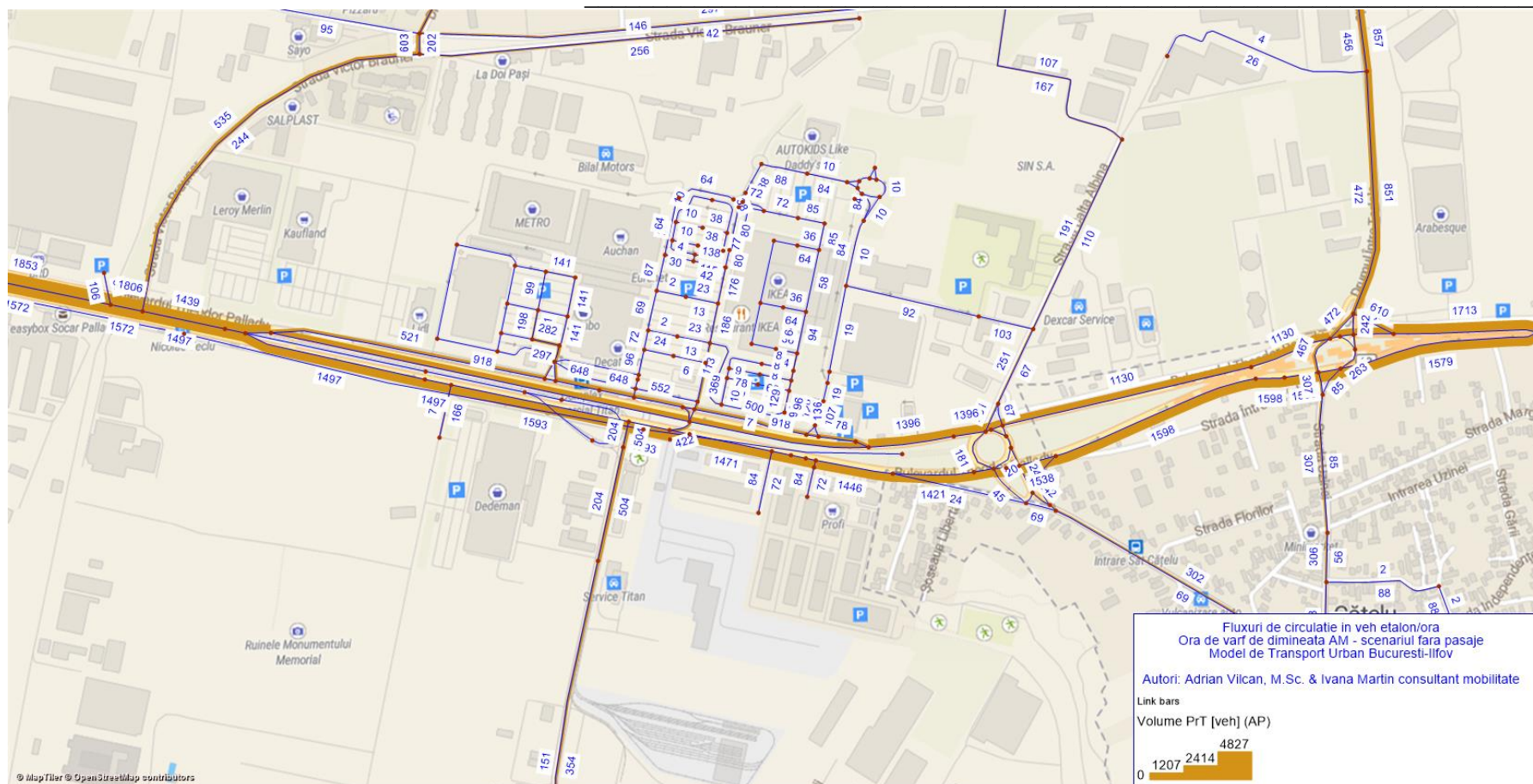
Fig. 32 – Debite de trafic - situația fără pasaje, ora de vârf de AM - veh/ora, detaliu Vest
