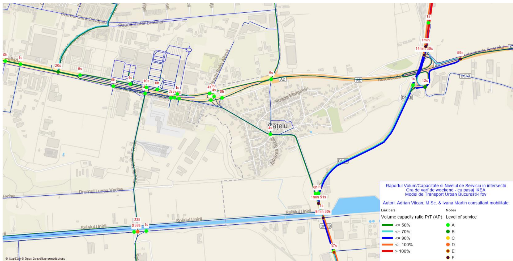
Fig. 76 – Întârzieri și Nivelul de Serviciu în intersecții - Raportul Volum/Capacitate pe bară dintre intersecții - scenariul cu pasaj IKEA, ora de vârf de sâmbătă, vedere de ansamblu
