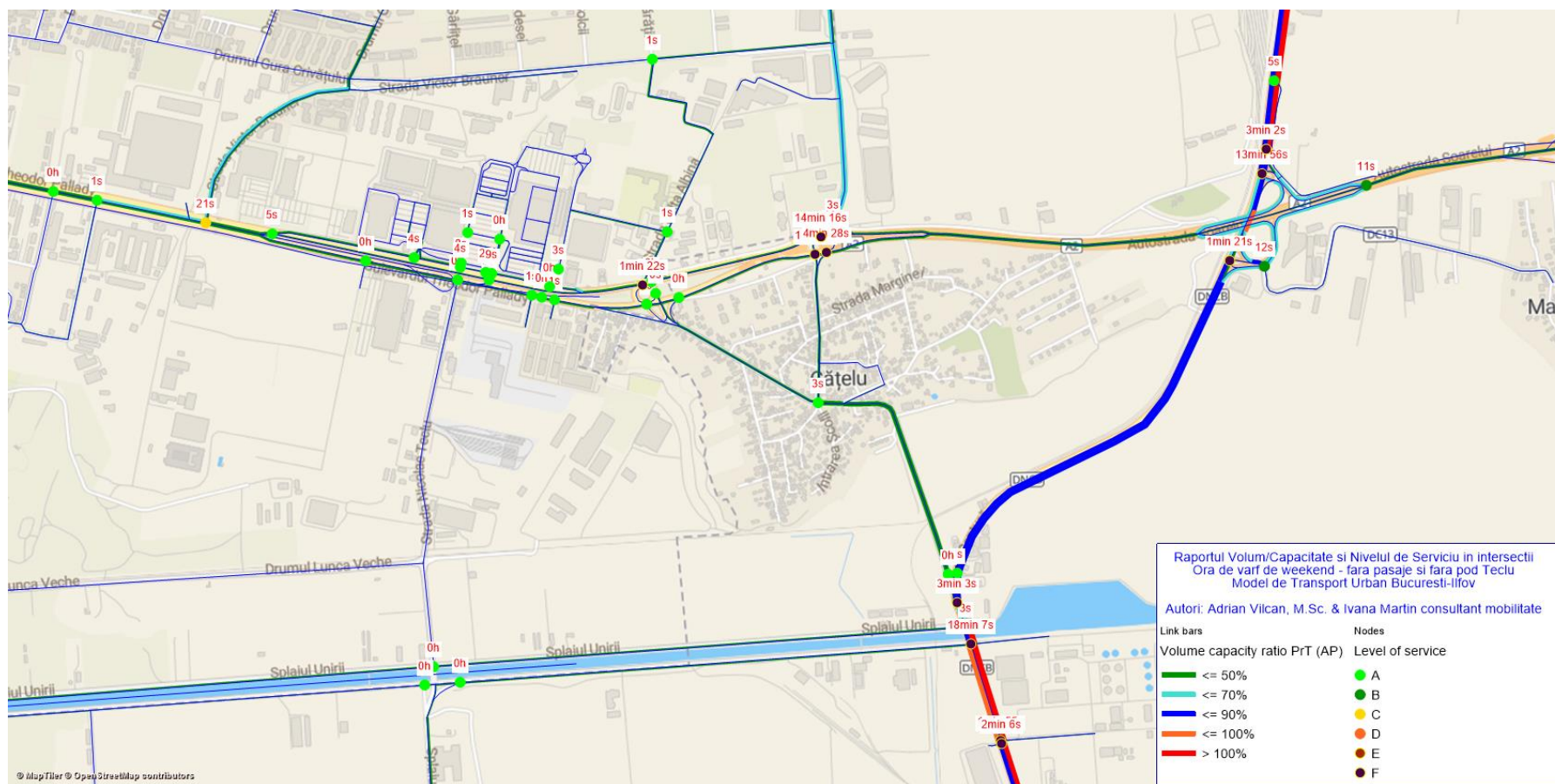
Fig. 64 – Întârzieri si Nivelul de Serviciu in intersectii - Raportul Volum/Capacitate pe bara dintre intersectii - situația fără pasaje fără pod Teclu, ora de vârf de sâmbătă, vedere de ansamblu
