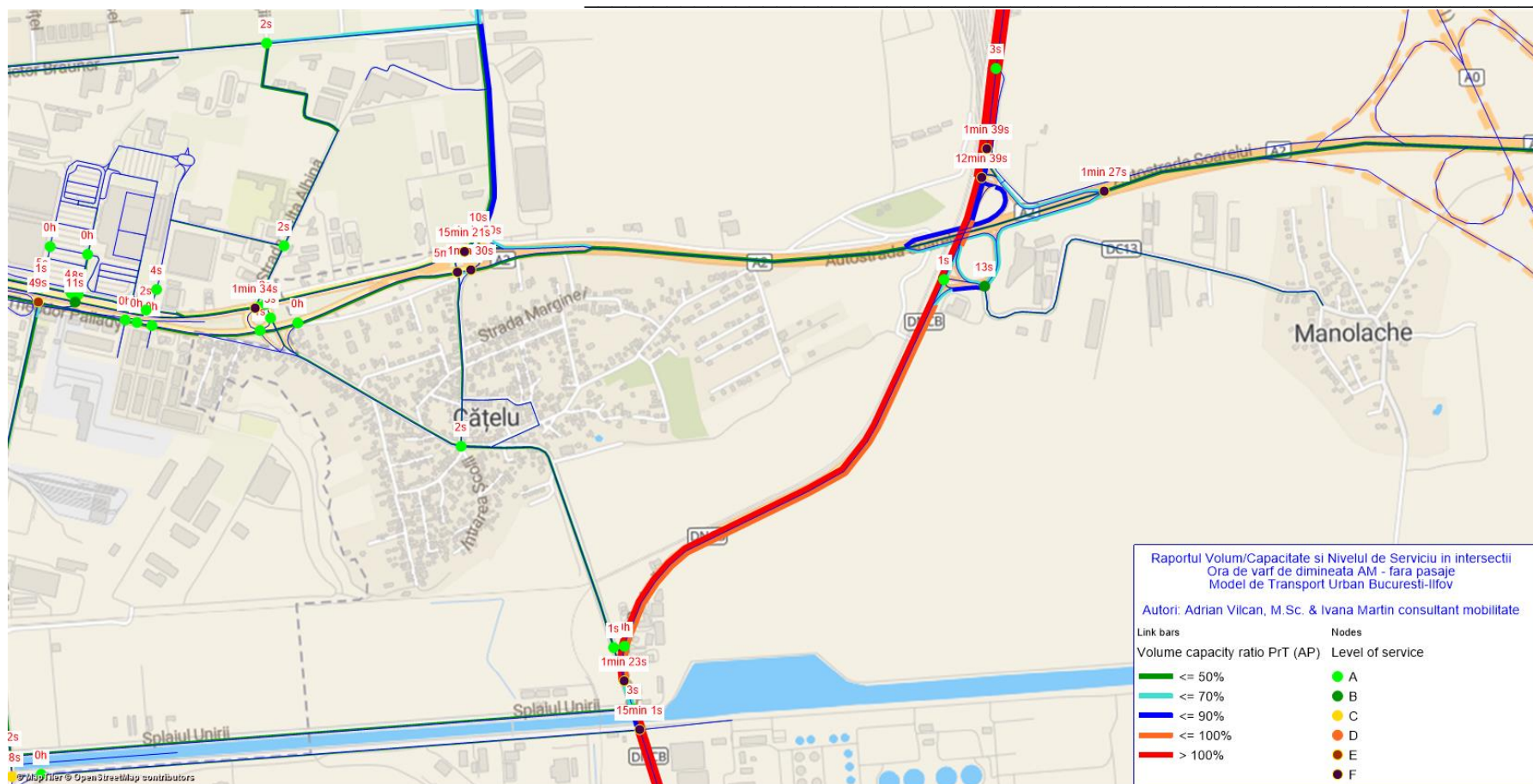
Fig. 36 – Întârzieri si Nivelul de Serviciu in intersectii - Raportul Volum/Capacitate pe bara dintre intersectii - situația fără pasaje, ora de vârf de dimineața AM, detaliu Est
