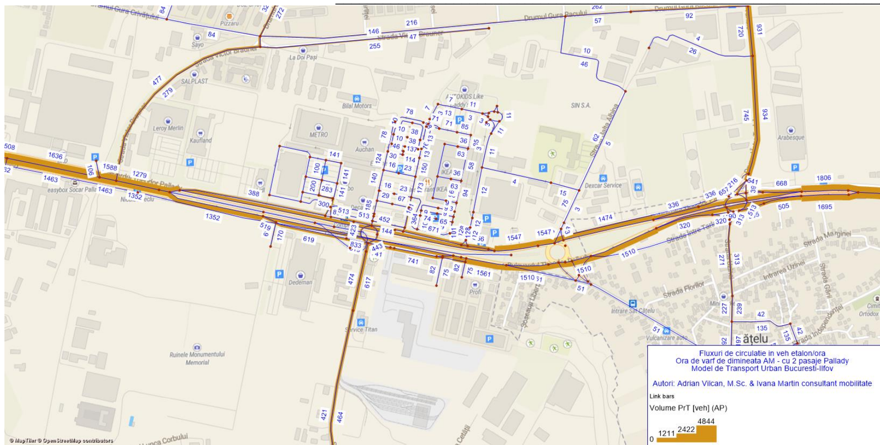
Fig. 8 – Debite de trafic - situația actuala de circulație ora de vârf de AM - vet/ora, detaliu Vest
