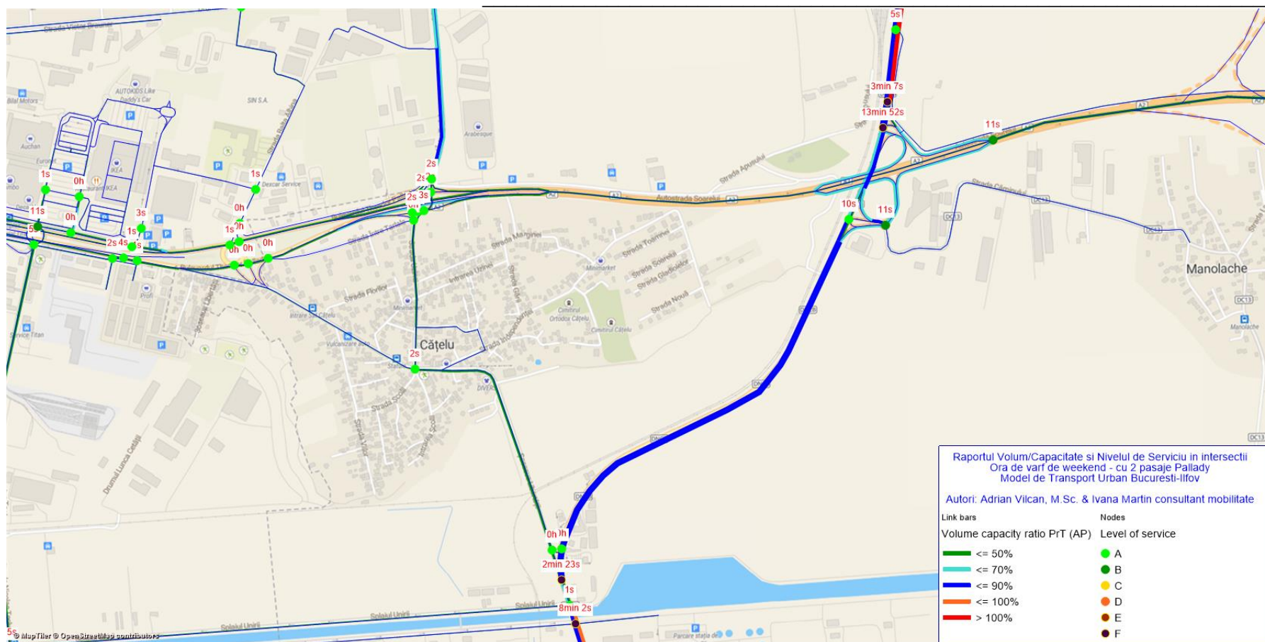
Fig. 60 – Întârzieri si Nivelul de Serviciu in intersectii - Raportul Volum/Capacitate pe bara dintre intersectii - situația actuala de circulație ora de vârf de sâmbătă, detaliu Est
