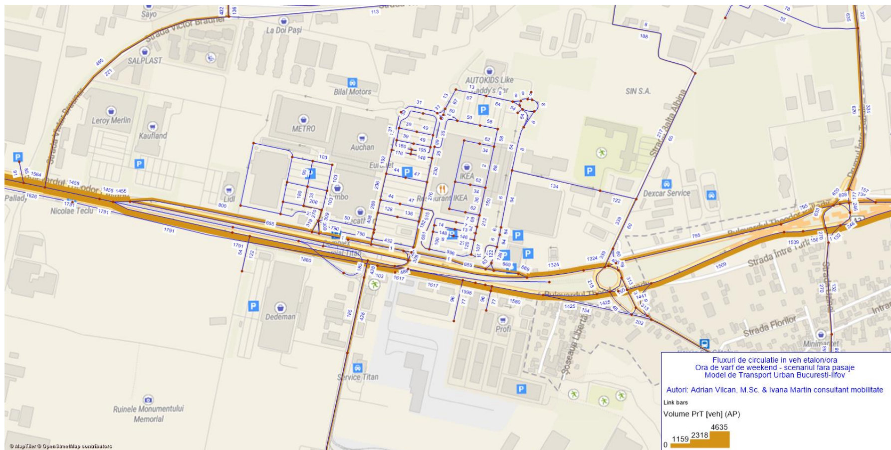
Fig. 68 – Debite de trafic - situația fără pasaje, ora de vârf de sâmbătă - veh/ora, detaliu Vest
