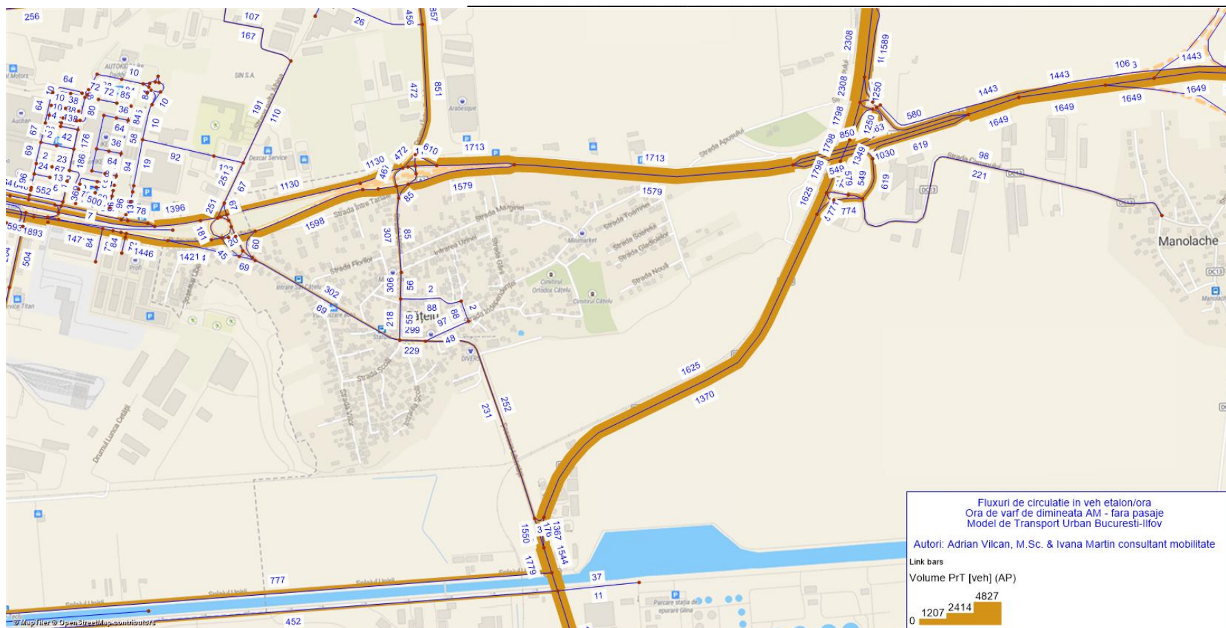
Fig. 33 – Debite de trafic - situația fără pasaje, ora de vârf de AM - veh/ora, detaliu Est
