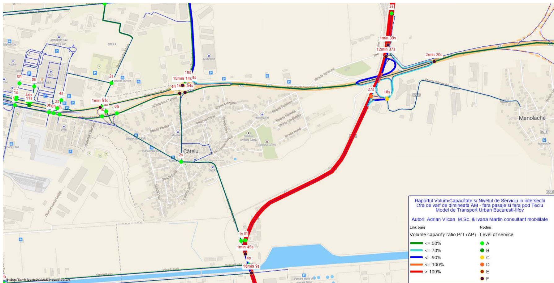
Fig. 24 – Întârzieri și Nivelul de Serviciu în intersecții - Raportul Volum/Capacitate pe bară dintre intersecții - situația fără pasaje fără pod Teclu, ora de vârf de dimineața AM, detaliu Est
