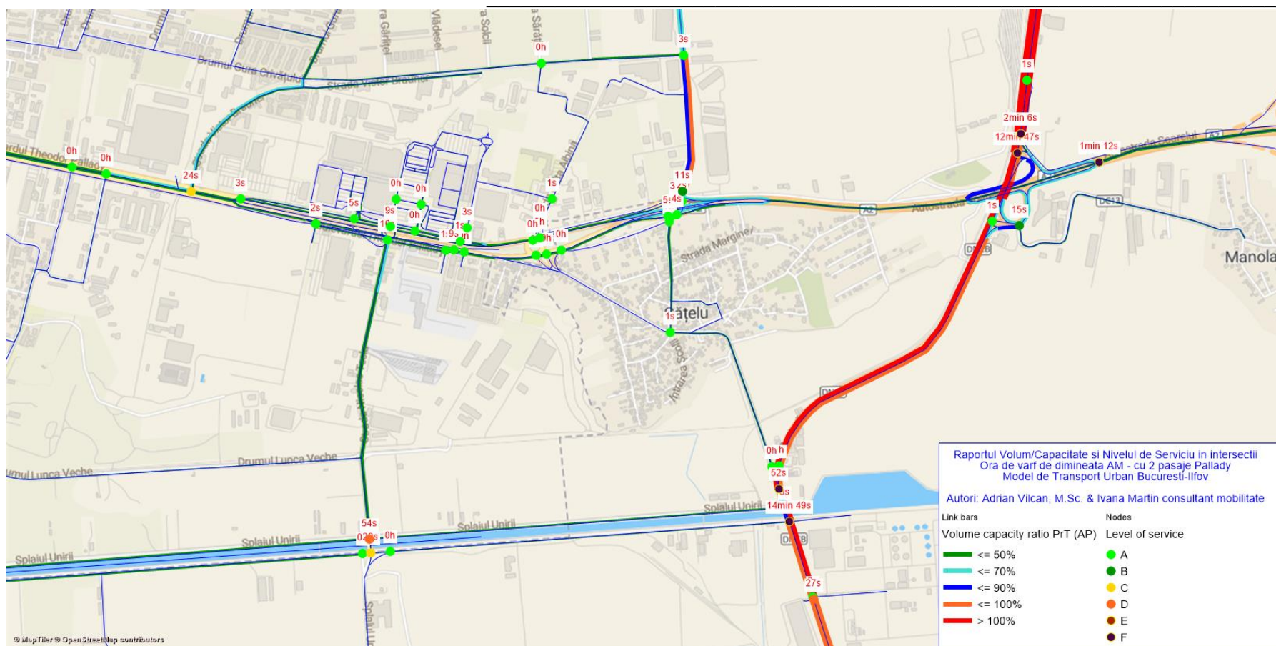
Fig. 10 – Întârzieri și Nivelul de Serviciu în intersecții - Raportul Volum/Capacitate pe bară dintre intersecții - situația actuală de circulație ora de vârf de dimineața AM, vedere de ansamblu
