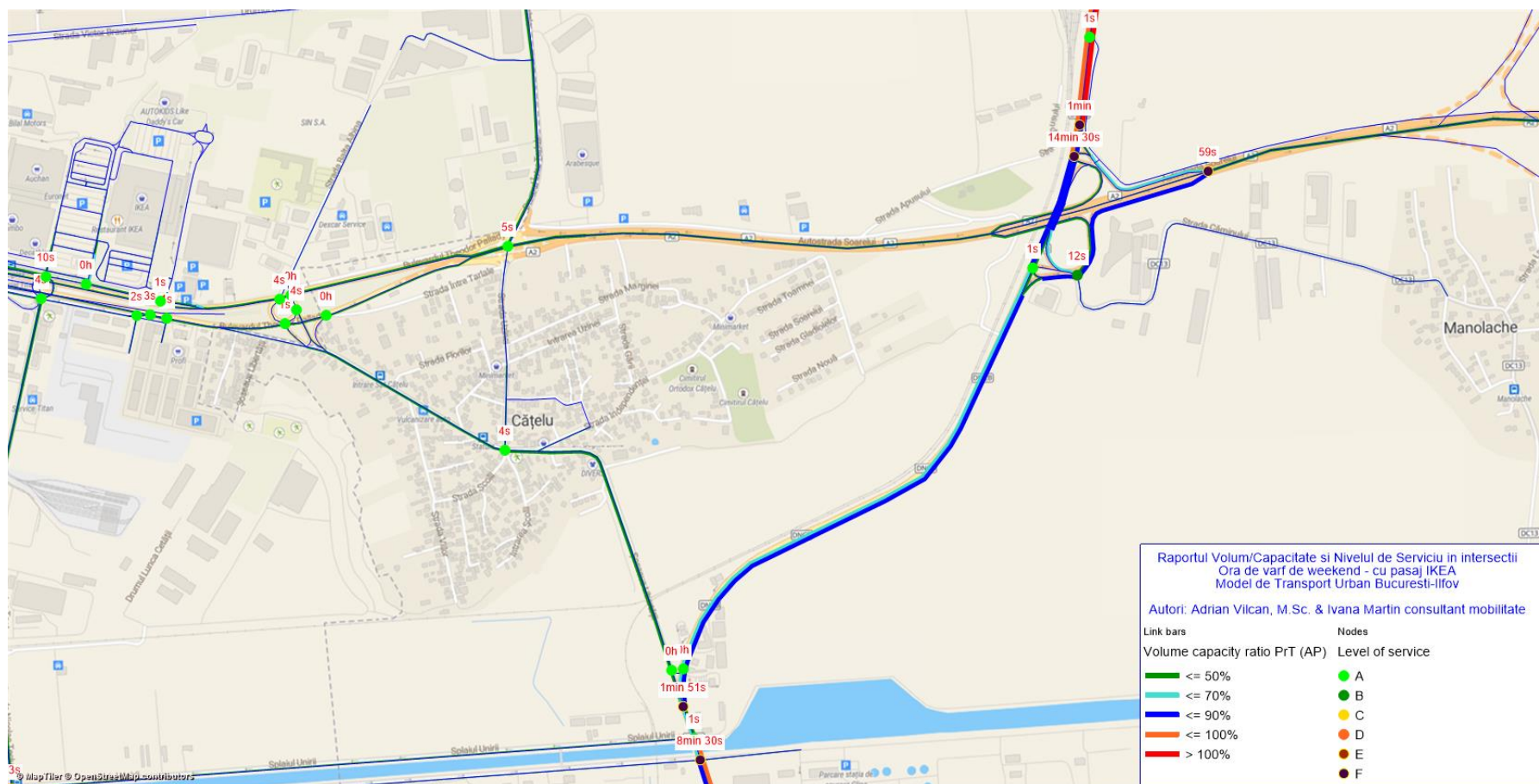
Fig. 78 – Întârzieri și Nivelul de Serviciu în intersecții - Raportul Volum/Capacitate pe bara dintre intersecții - scenariul cu pasaj IKEA, ora de vârf de sâmbătă, detaliu Est
