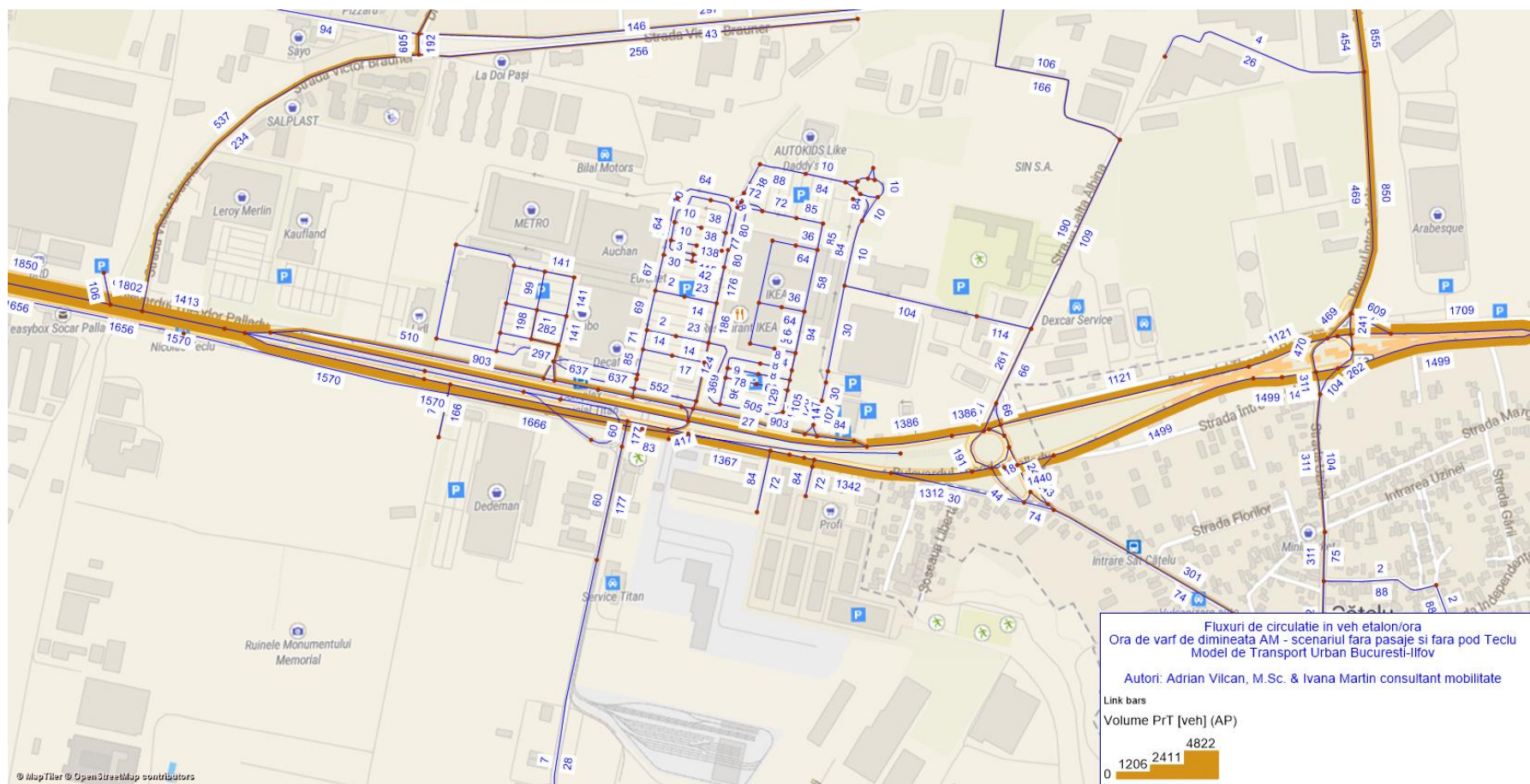
Fig. 20 – Debite de trafic - situația fără pasaje fără pod Teclu, ora de vârf de AM - veh/ora, detaliu Vest
