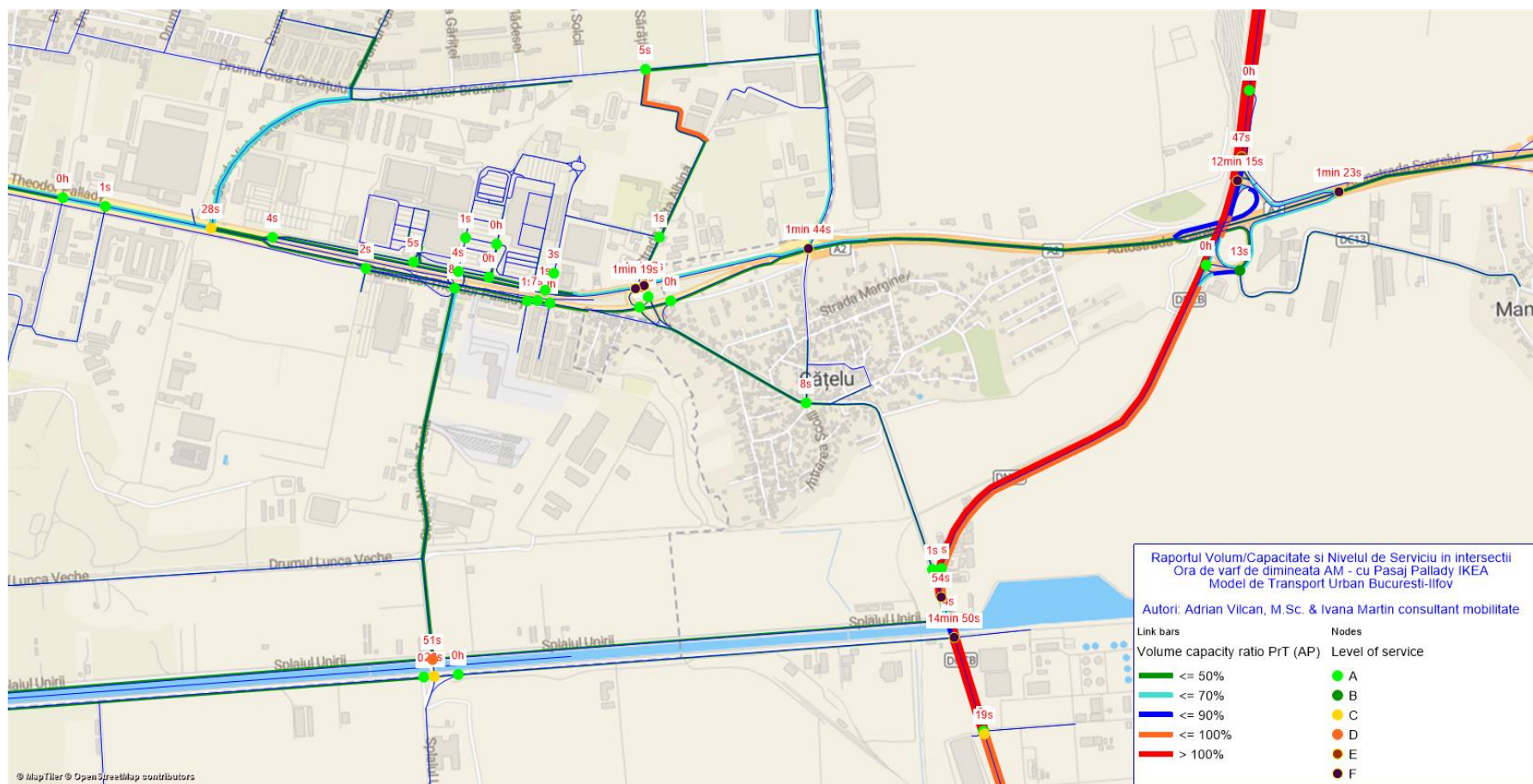
Fig. 46 – Întârzieri și Nivelul de Serviciu în intersecții - Raportul Volum/Capacitate pe bară dintre intersecții - scenariul cu pasaj IKEA, ora de vârf de dimineața AM, vedere de ansamblu
