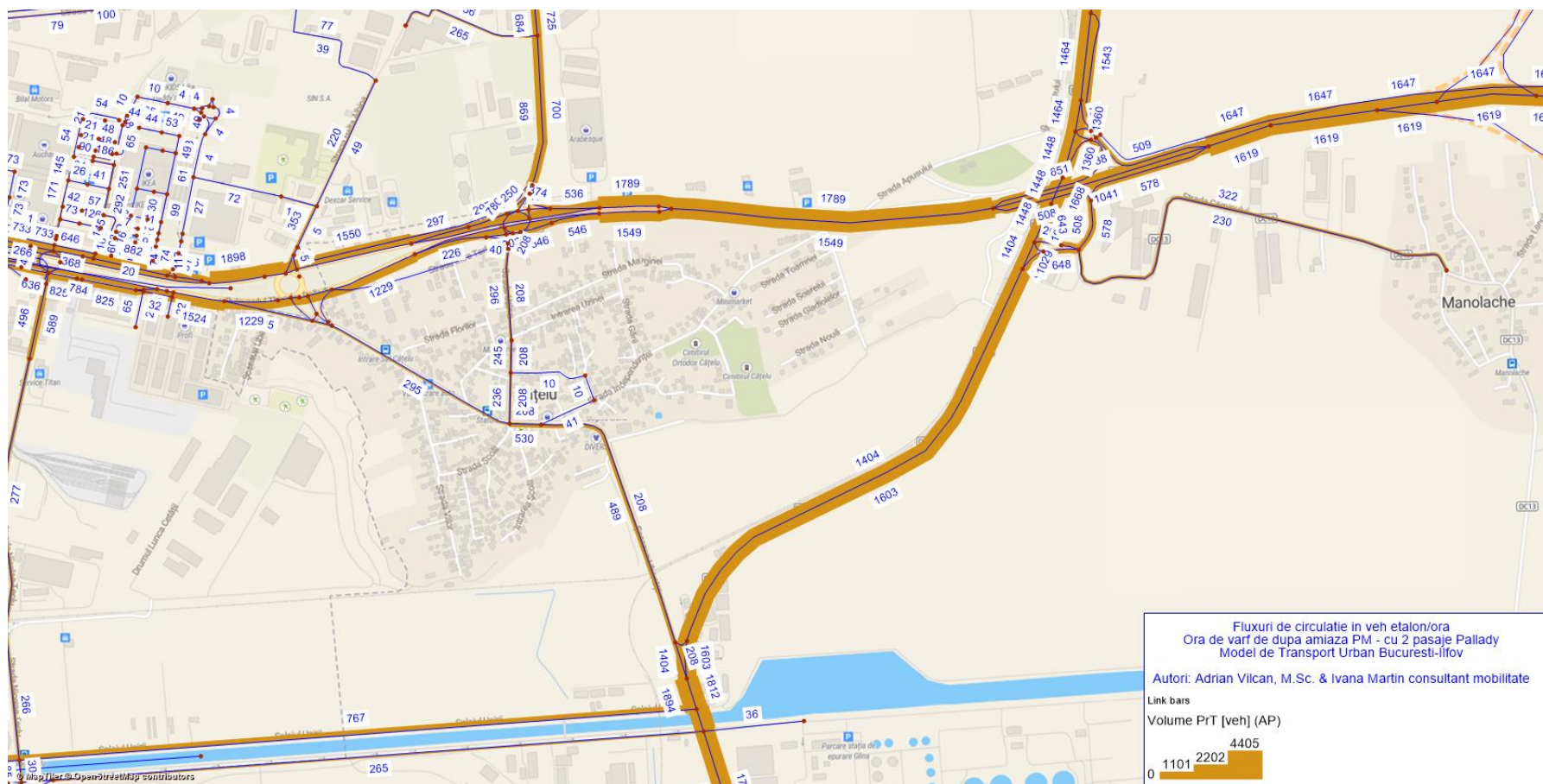
Fig. 15 – Debite de trafic - situația actuala de circulație ora de vârf de PM - veh/ora, detaliu Est
