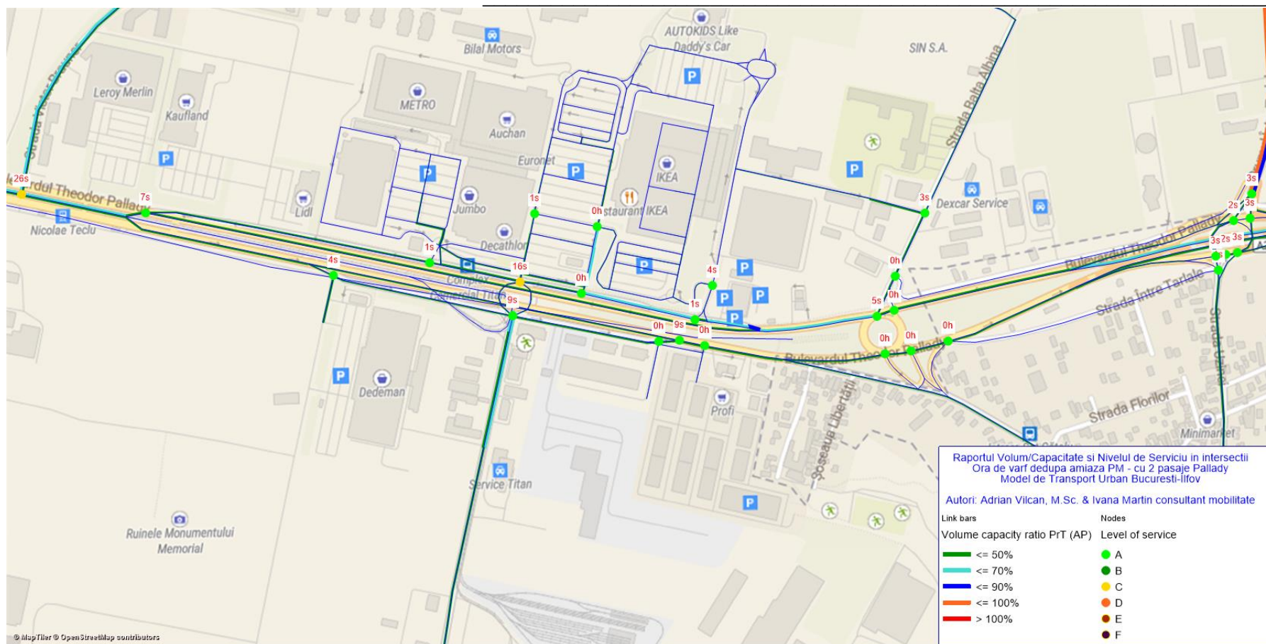
Fig. 17 – Întârzieri și Nivelul de Serviciu în intersecții - Raportul Volum/Capacitate pe bară dintre intersecții - situația actuală de circulație ora de vârf de după amiaza PM, detaliu Vest
