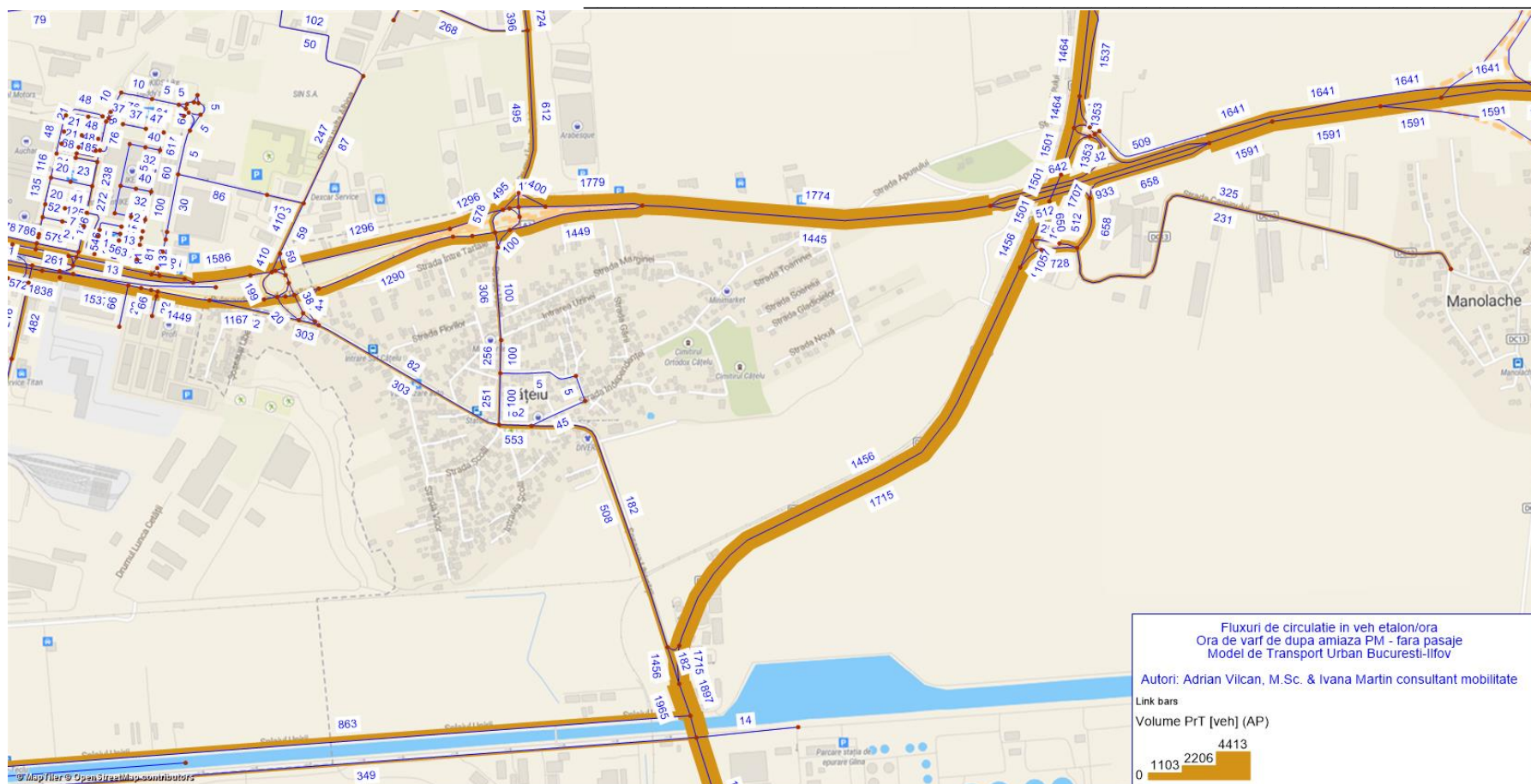
Fig. 39 – Debite de trafic - situația fără pasaje, ora de vârf de PM - veh/ora, detaliu Est
