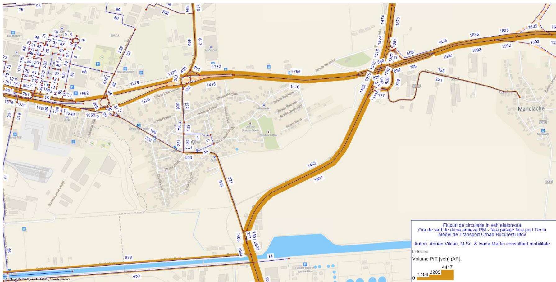
Fig. 27 – Debite de trafic - situația fără pasaje fără pod Teclu, ora de vârf de PM - vet/ora, detaliu Est
