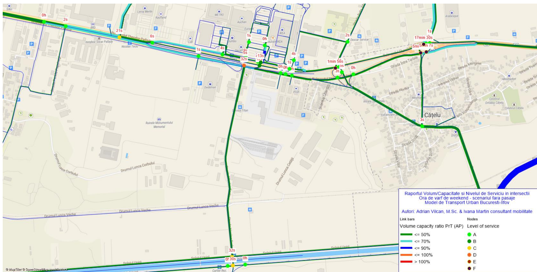
Fig. 71 – Întârzieri si Nivelul de Serviciu in intersectii - Raportul Volum/Capacitate pe bara dintre intersectii - situația fără pasaje, ora de vârf de sâmbătă, detaliu Vest
