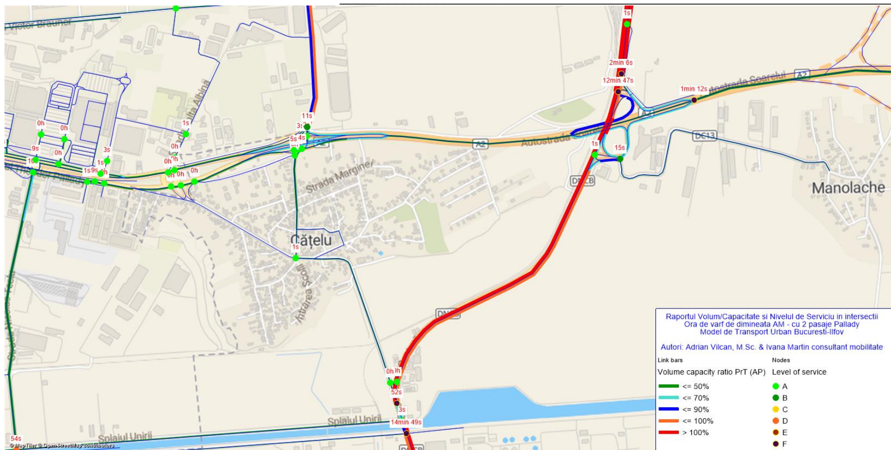
Fig. 12 – Întârzieri si Nivelul de Serviciu in intersectii - Raportul Volum/Capacitate pe bara dintre intersectii - situația actuala de circulație ora de vârf de dimineața AM, detaliu Est
