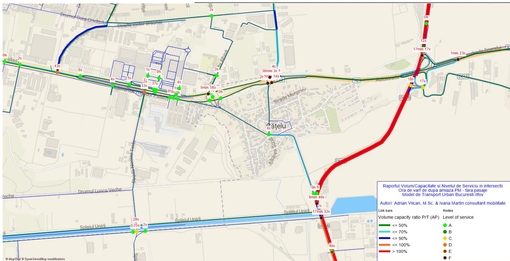
Fig. 40 – Întârzieri și Nivelul de Serviciu în intersecții - Raportul Volum/Capacitate pe bară dintre intersecții - situația fără pasaje, ora de vârf de după amiaza PM, vedere de ansamblu
