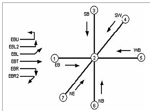
Fig. 80 – Codificarea direcțiilor de deplasare în intersecție
