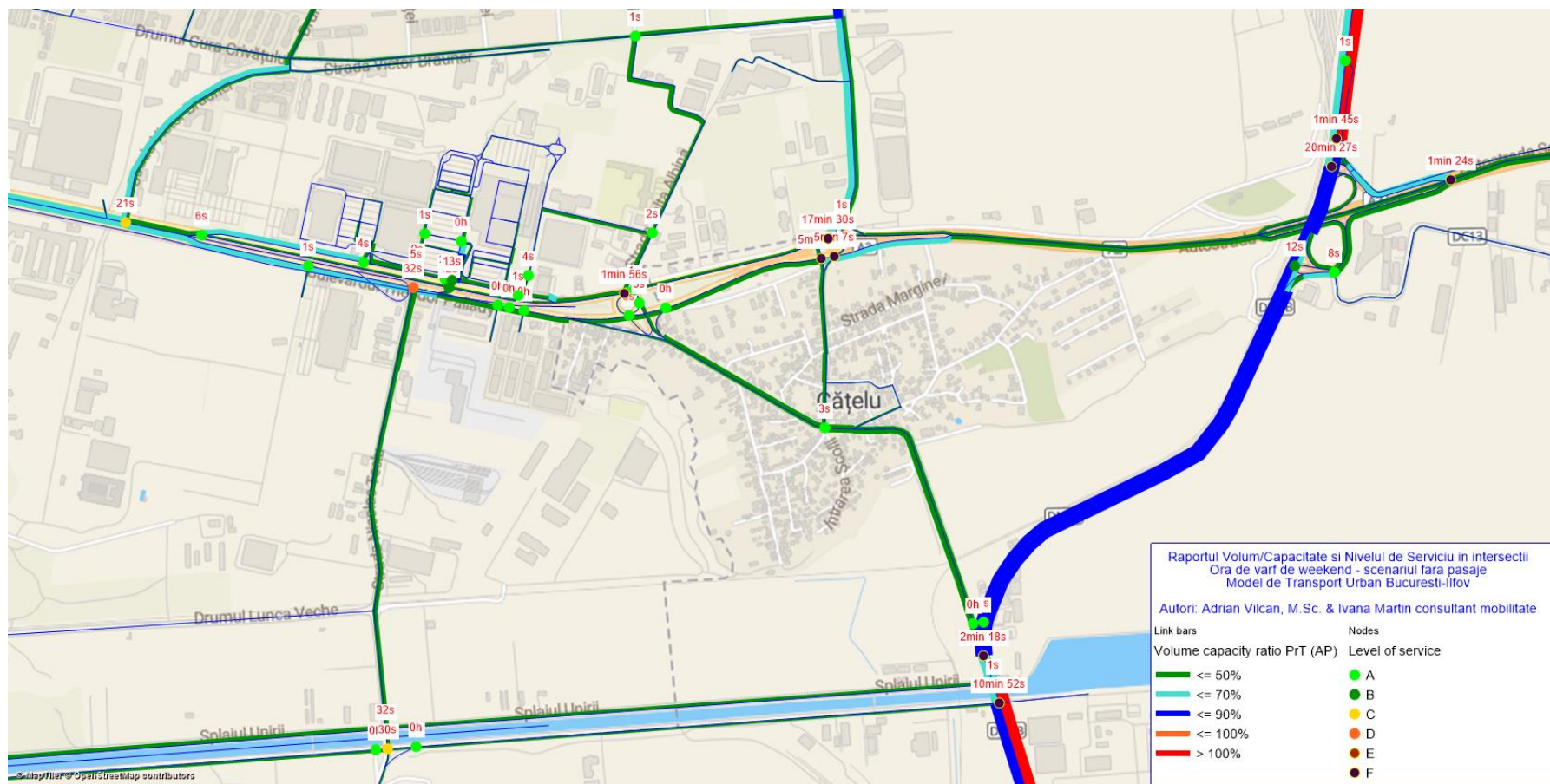
Fig. 70 – Întârzieri si Nivelul de Serviciu in intersectii - Raportul Volum/Capacitate pe bara dintre intersectii - situația fără pasaje, ora de vârf de sâmbătă, vedere de ansamblu
