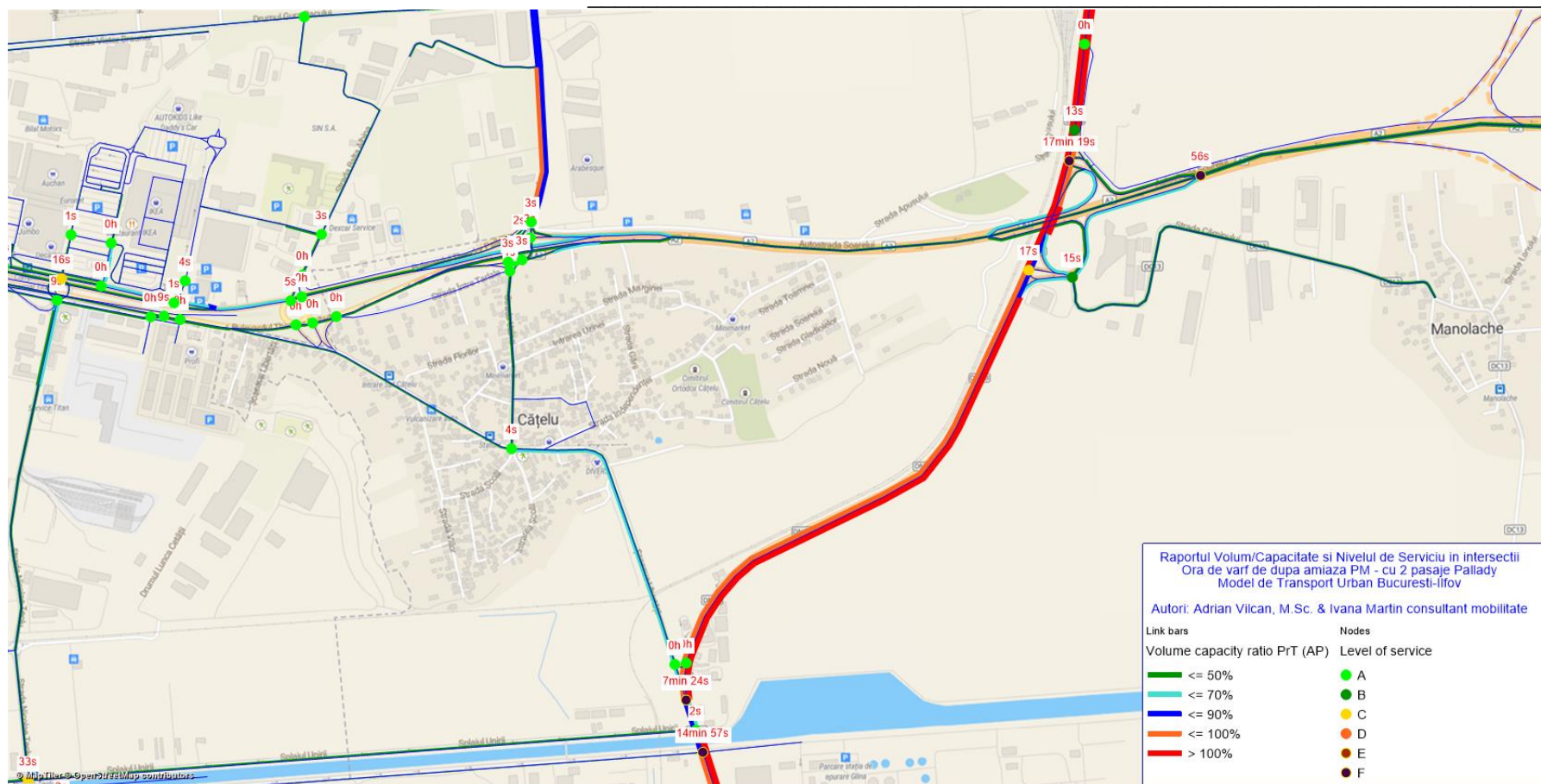
Fig. 18 – Întârzieri și Nivelul de Serviciu în intersecții - Raportul Volum/Capacitate pe bară dintre intersecții - situația actuală de circulație ora de vârf de după amiaza PM, detaliu Est
